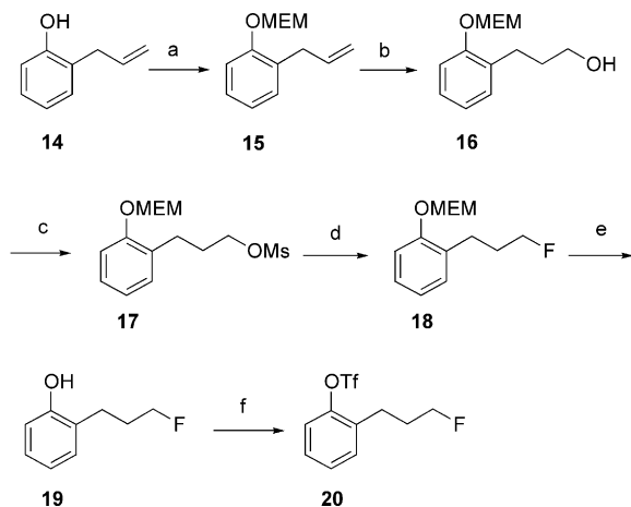
Scheme 3. (a) MEMCl, NaH, THF, 0 °C to reflux, 1 h, 82%; (b) borane–THF complex, H 2 O 2 , 4 N NaOH, THF, 0 °C, 1 h, 48%; (c) MsCl, Et 3 N, CH 2 Cl 2 , 0 °C, 20 min, 56%; (d) n -Bu 4 NF·xH 2 O, CH 3 CN, 110 °C, 30 min, 74%; (e) concd HCl, MeOH, 60 °C, 1 h, 90%; (f) Tf 2 O, 2,6-lutidine, CH 2 Cl 2 , 0 °C to rt, N 2 , 30 min, 82%.
