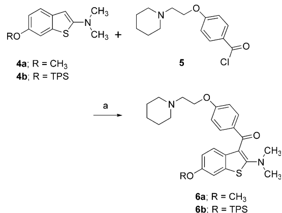
Scheme 1. (a) Chlorobenzene, 100 °C, 9 h, 6a : 64%; 6b : 68%.
